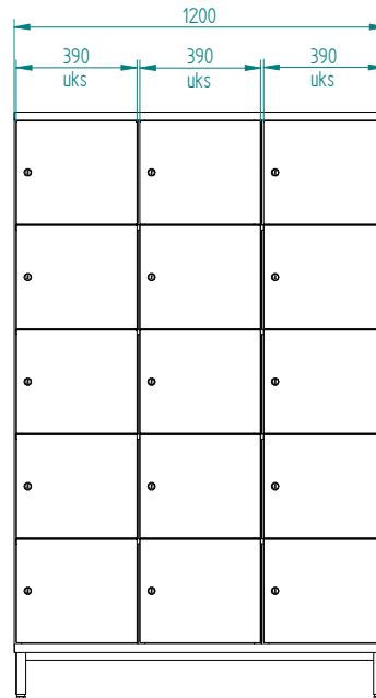
SK5 3/400
