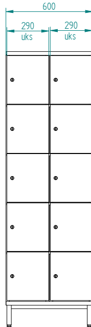
SK5 2/300
