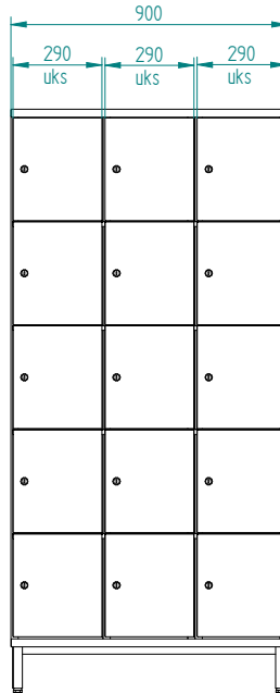
SK5 3/300
