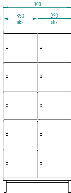
SK5 2/400
